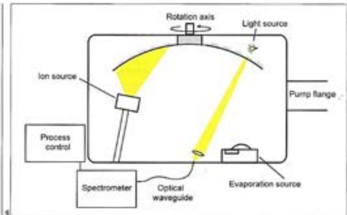
Figure 1 : Schéma d'une chambre d'application à vaporisation par faisceau d'électrons ionique et à surveillance optique à large bande de l'épaisseur des couches.
