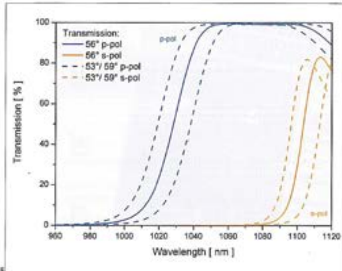
Figure 3 : Courbe de transmission du polarisateur en couche mince à large bande (TFPB) pour une longueur d'onde centrale de 1064 nm.
