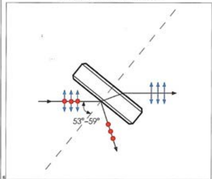
Figure 2 : Un polarisateur en couche mince est inséré en dessous de l'angle de Brewster d'environ 56^\circ . Alors que la lumière à polarisation p est transmise, la partie à polarisation s est réfléchie, et donc déviée de 112^\circ .
