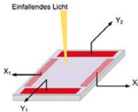
Schematischer Aufbau eines Duo-Lateralen PSDs
