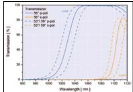
▲ Figure 3 : Courbe de transmission du polarisateur en couche mince à large bande (TFPB) pour une longueur d'onde centrale de 1064 nm.
