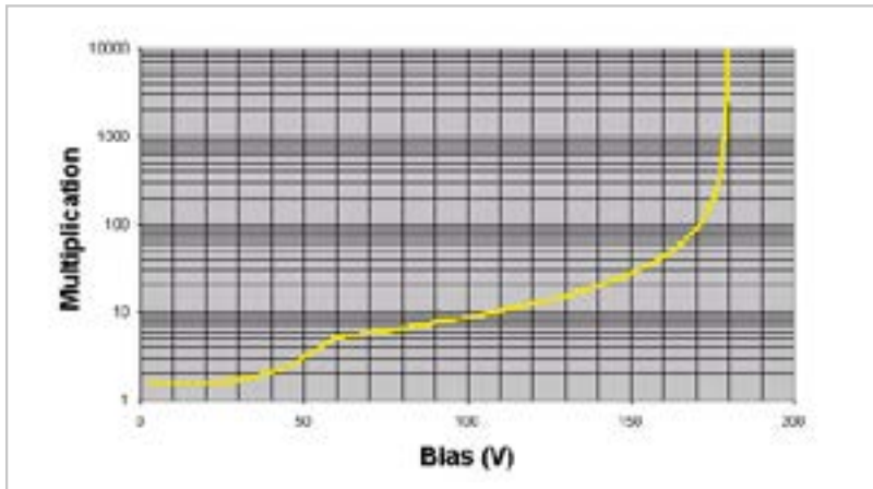
Abb. 1: Typische Verstärkung vs. Betriebsspannung (0,5 mm APD)
