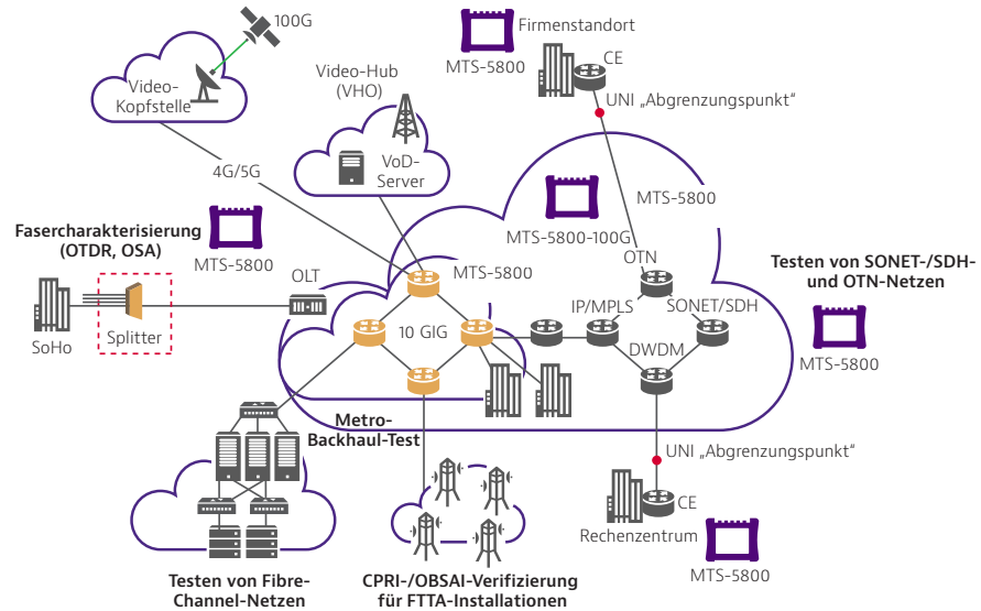
Abbildung 1: Einsatzmöglichkeiten des MTS-5800 in einem Carrier-Ethernet-Netz
