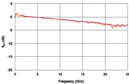
NIR-MX800-LN-20: 30 ps Square Pulse
