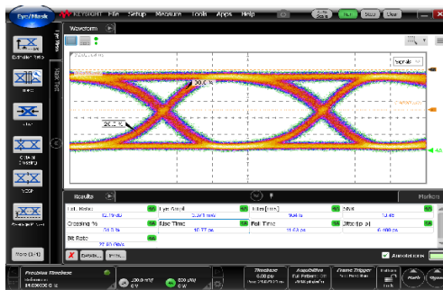
28 Gb/s OOK-NRZ eye diagram
