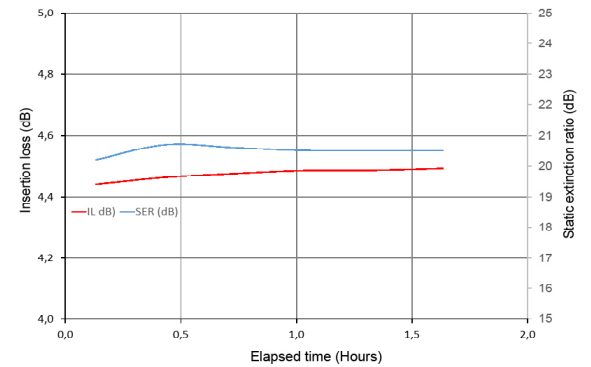
IL & SER stability @25° C and Pin = 300 mW
