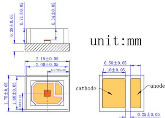
VD-0940I-050W-3A-3A0 (Channel array 1X1, Substrate CuAg, Package 2016)
