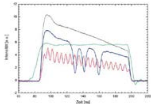
Bild 9: Absorptionslinien (blau) des ^{15}NH_3 und Interferenzen eines Germanium-Etalons (rot). Linienpositionen von rechts nach links ( cm^{-1} : 882,85; 883,01; 883,11 ( I_{amp} = 5,6 A ; f = 8 kHz ; t_{puls} = 120 ns ). Zum Vergleich sind das reine Lasersignal (schwarz) und der Strompuls des Treibers (grün) dargestellt.
