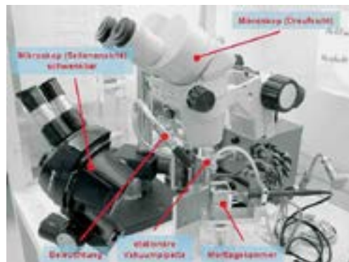
Bild 3: Workstation zur Verarbeitung von Quantenkaskadenlasern in Standardgehäuse
