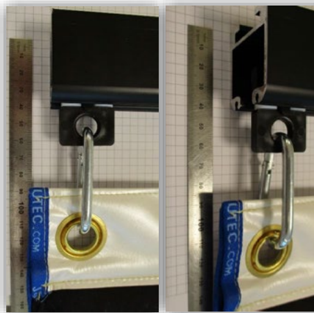
Schienenprofil
