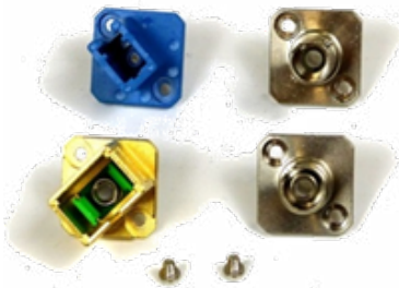
Optische Adapter (BN 2155) für Laserquellen
