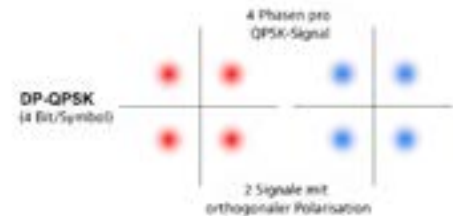
Abbildung 3: Signal beim DP-QPSK-Modulationsverfahren
