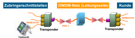
Abbildung 1: Transponder-Konfiguration
