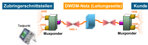
Abbildung 2: Muxponder-Konfiguration
