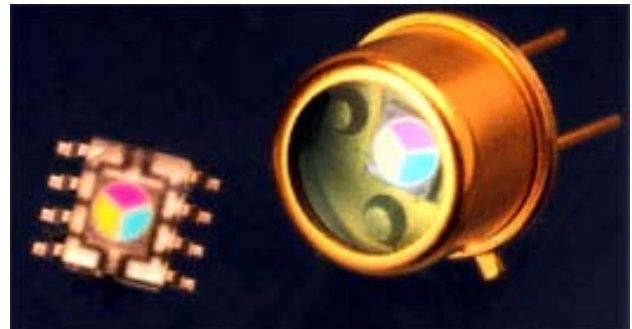
Bild 3: Drei-Elemente-Farbsensor-ICs im SMD und TO-5-Gehäuse
