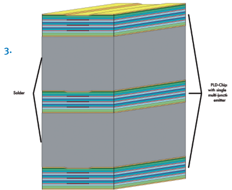
Verschiedene Aufbauten von PLDs: 1. Einzelemitter, 2. Multi-Junction Chip mit drei Emittern, 3. Stapelaufbau aus drei Multi-Junction Chips
