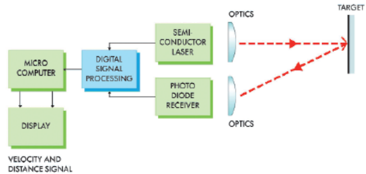
Funktionsprinzip der Pulslaufzeit
