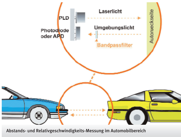
Funktionsprinzip der Pulslaufzeit
