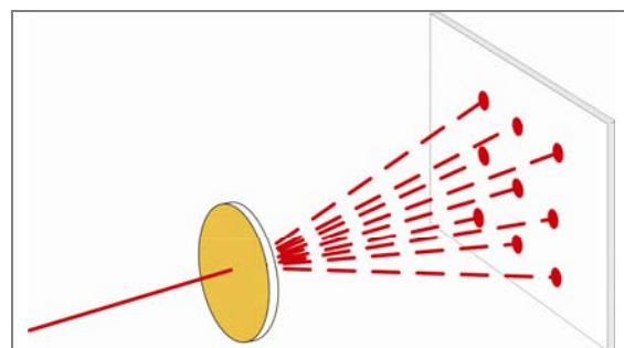
Abb. 2: Zweidimensionale DOEs führen zu einem Punktraster. In der Abbildung sehen Sie ein 3 x 3 Element welches neun Punkte in der Beobachtungsebene erzeugt.
