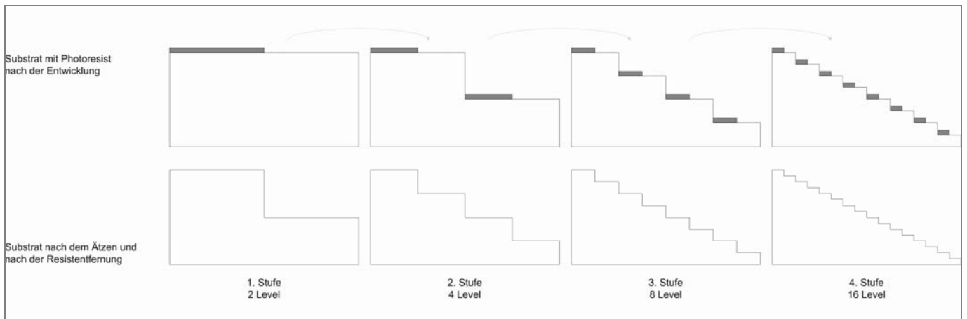
Abb. 6: Werden die Prozessschritte zur Erstellung eines DOEs mehrfach wiederholt, so werden die Stufen, die in das DOE geätzt werden immer kleiner, das Ergebnis damit immer genauer. Das Ergebnis der Stufenverfeinerung sehen Sie deutlich in der Abb. 7.
