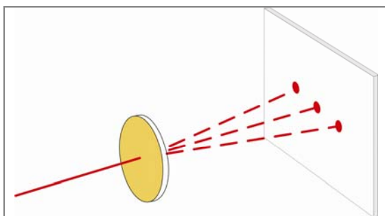
Abb. 1: 1 x 3 Matrix in schematischer Darstellung- Eine 1 x 3 Matrix erzeugt in der Beobachtungsebene drei Punkte auf einer Linie
