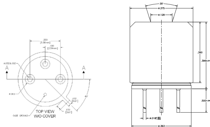
Figure 24. TSM package, 35 deg FOV (MD-0005, MD-0007).
