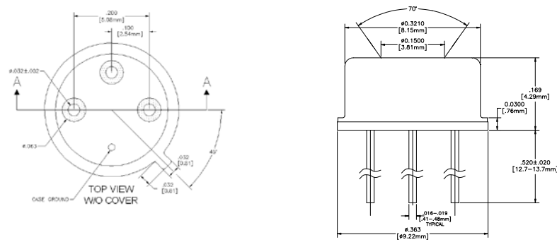
Figure 23. TSM package, 70 deg FOV (MD-0003, MD-0006, MD-0008).
