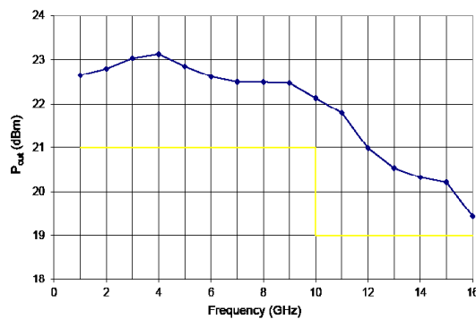
P1 dB Parameter Curve
